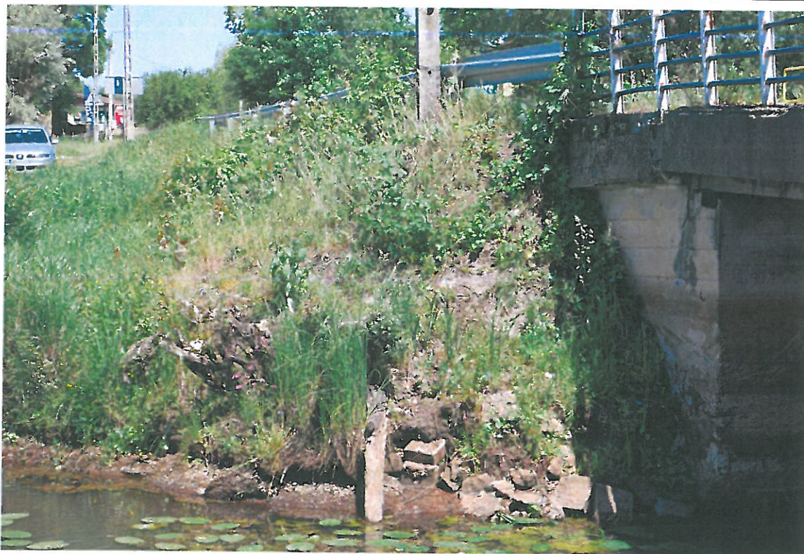
Fot. 5. Wegetacja roślin oraz zanieczyszczenia stożka spowodowane brakiem systematycznych prac utrzymaniowych (stożek od strony północnej – widok od strony dolnej wody)
